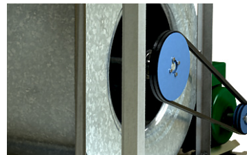
Detalle de los componentes de la transmisión.
